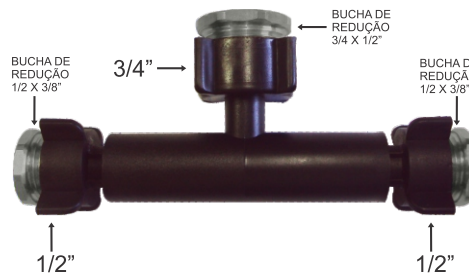
TEE P/ MISTURADOR UNIVERSAL
