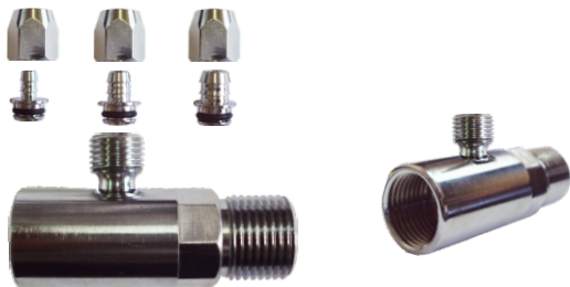
ADAPTADOR PARA FILTRO 1/2 SAÍDA MANGUEIRA C/ ESPIGA UNIVERSAL
